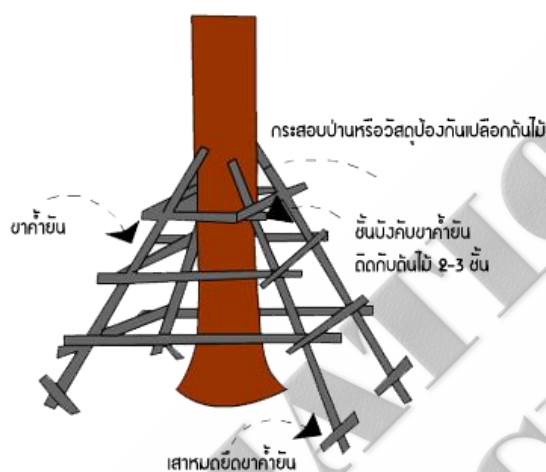
ภาพประกอบ 35 การค้ำยันแบบใช้แรงดึง
